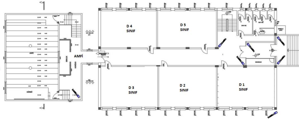
SAĞLIK HİZMETLERİ MESLEK YÜKSEK OKULU 1. KAT PLANI ÖLÇEK:1 / 50
