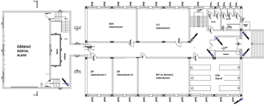
SAĞLIK HİZMETLERİ MESLEK YÜKSEK OKULU ZEMİN KAT PLANI ÖLÇEK:1 / 50
